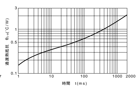
θja-t特性
