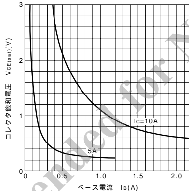
VCE(sat)-Ib特性 (代表例)
