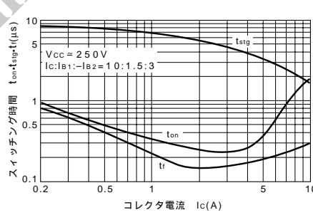
ton•tstg•tf-Ic特性 (代表例)
