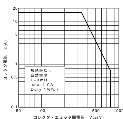
逆バイアスASO曲線
