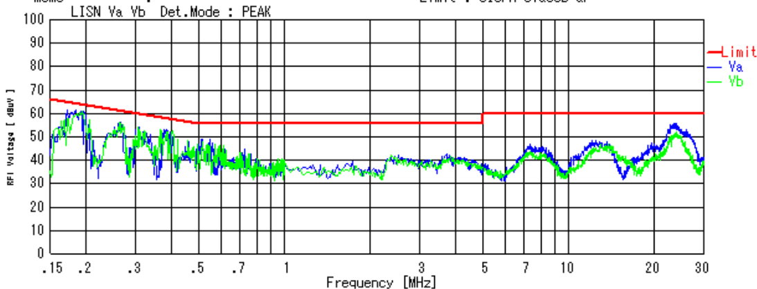
図20 雑音端子電圧
