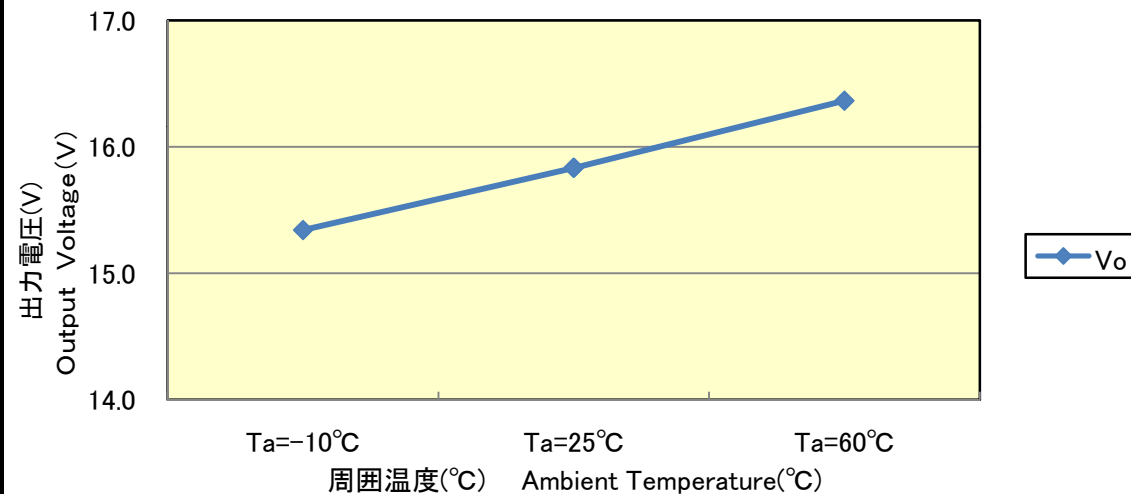
図11 過電圧特性(温度に対して) Fig.11 Over Voltage Protection Characteristics (vs Temperature)
