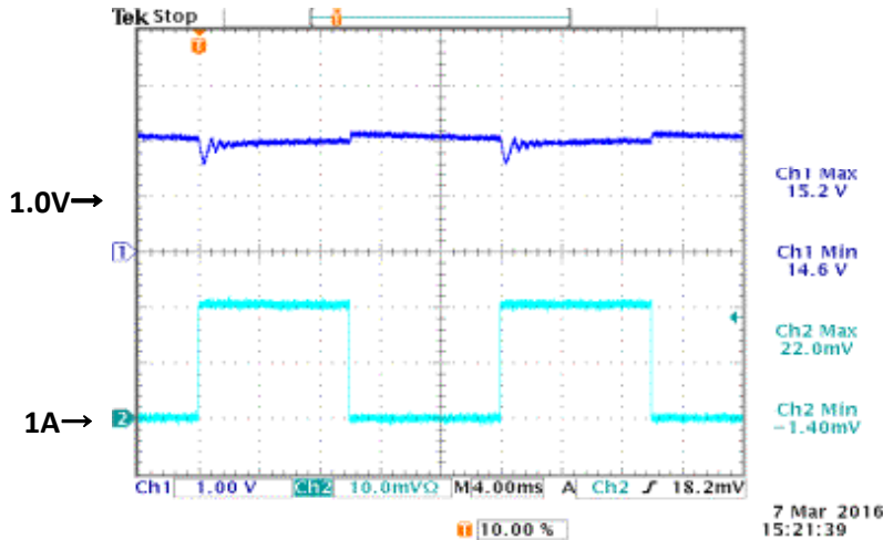
図14 ダイナミック時の負荷波形 Fig.14 Dynamic Load Waveform
