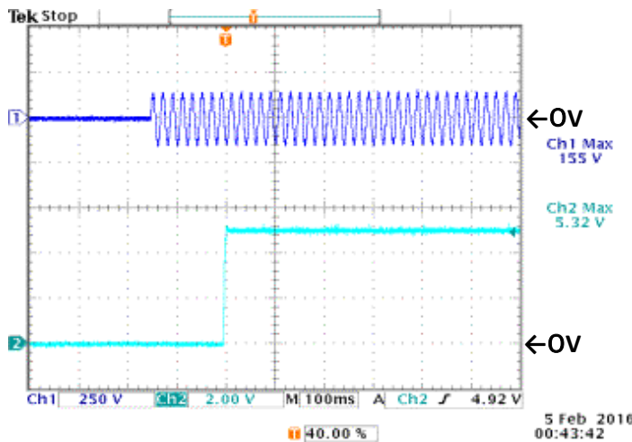
図15 出力電圧立上り波形 Fig.15 Output Voltage Rising Waveform
