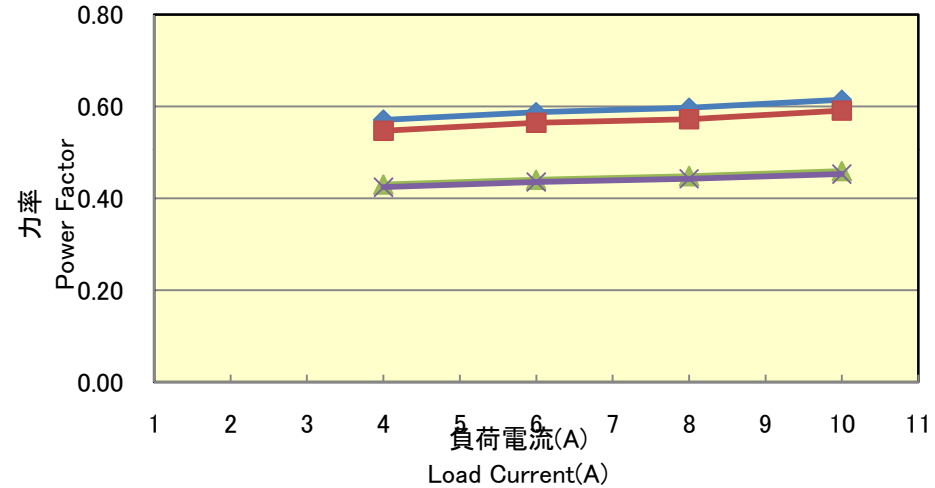
図2 力率特性(負荷電流に対して) Fig.2 Power Factor Characteristics (vs Load Current)
