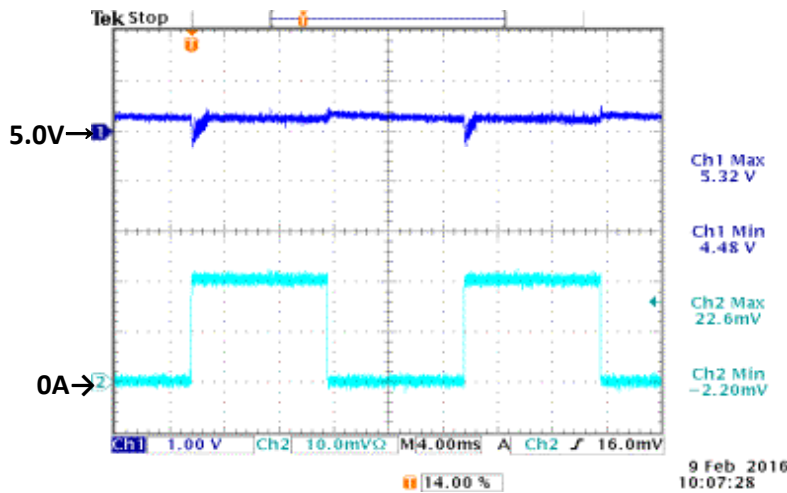
図14 ダイナミック時の負荷波形 Fig.14 Dynamic Load Waveform
