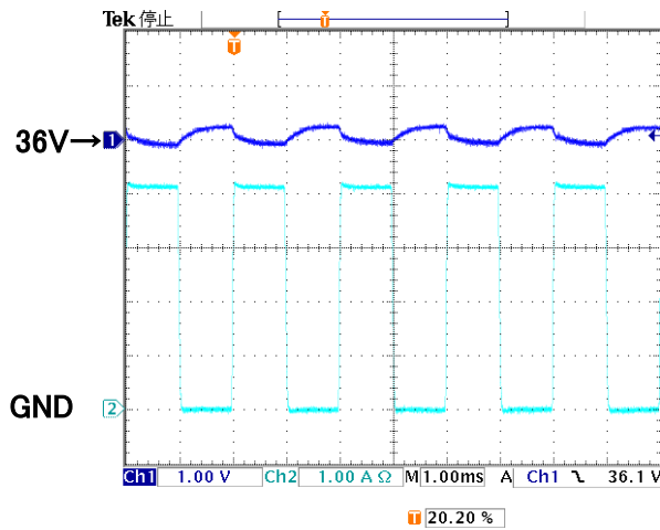
図13 タイミング時の負荷波形 Fig.13 Dynamic Load Waveform
