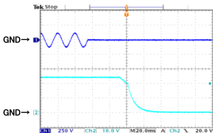
図15 出力電圧立下り波形 Fig.15 Output Voltage Falling Waveform
