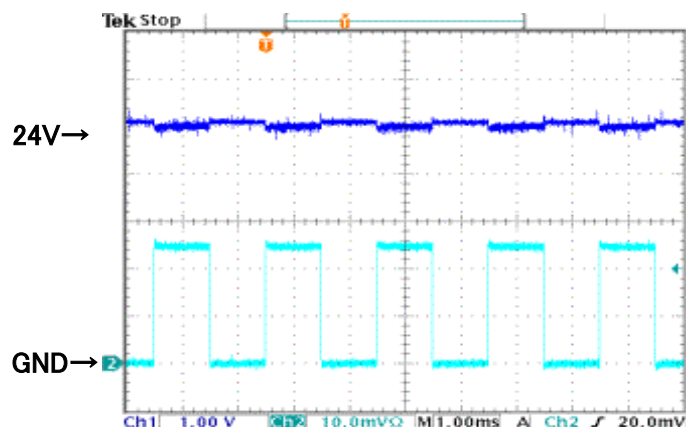
図13 タイミング時の負荷波形 Fig.13 Dynamic Load Waveform
