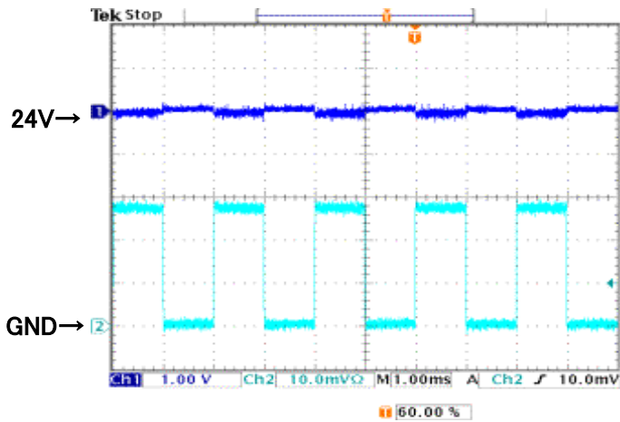
図13 タイミング時の負荷波形 Fig.13 Dynamic Load Waveform
