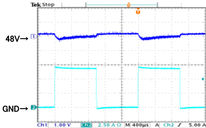
図13 ダイミク時の負荷波形 Fig.13 Dynamic Load Waveform
