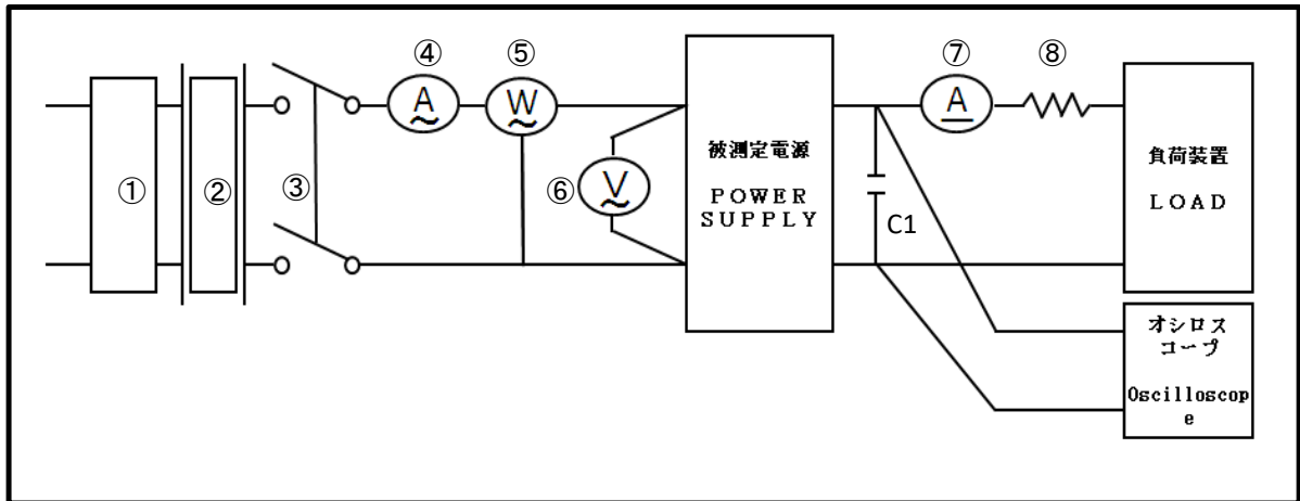
試験回路図 Test Circuit
