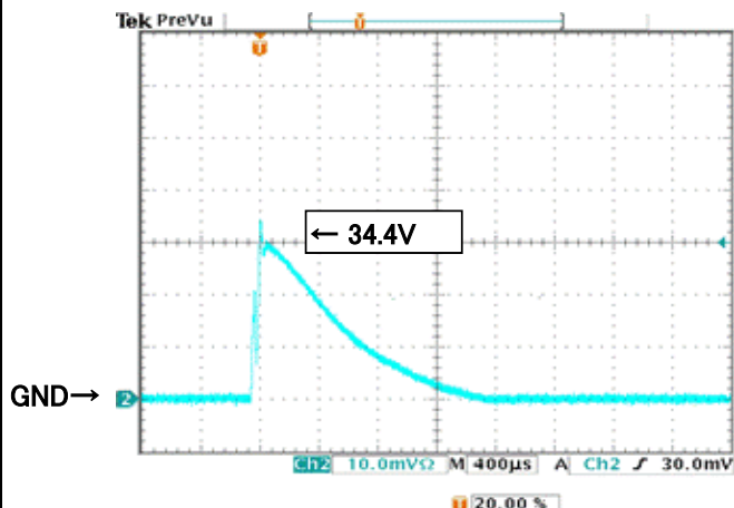
図17 過電圧波形
