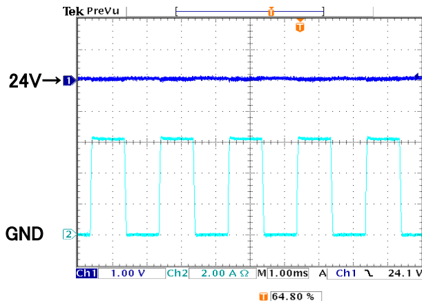
図13 ダイナミック時の負荷波形 Fig.13 Dynamic Load Waveform
