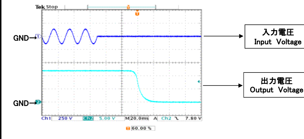
図15 出力電圧立下り波形 Fig.15 Output Voltage Falling Waveform
