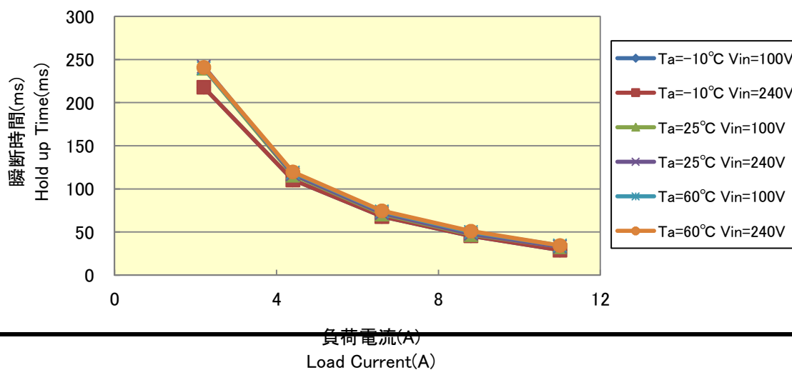
図12 入力瞬断時間(負荷電流に対して) Fig.12 Hold up time Characteristics (vs Load Current)
