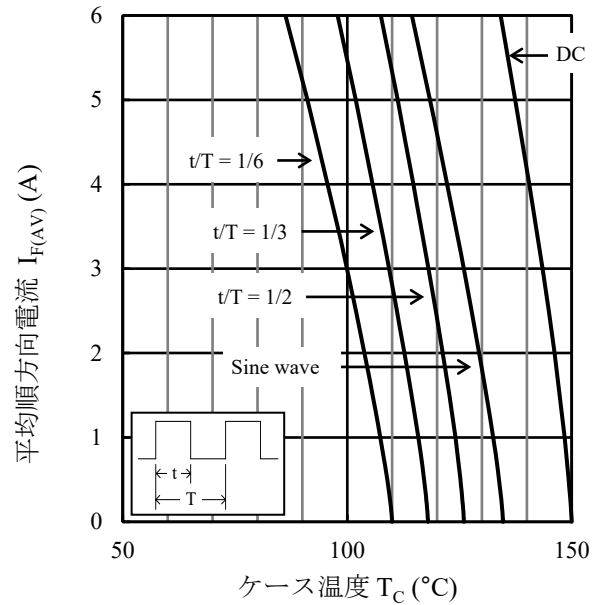
図2 I_{F(AV)} - T_C 特性 ( T_J = 150\text{ }^\circ\text{C} 、 V_R = 60\text{ V} )
