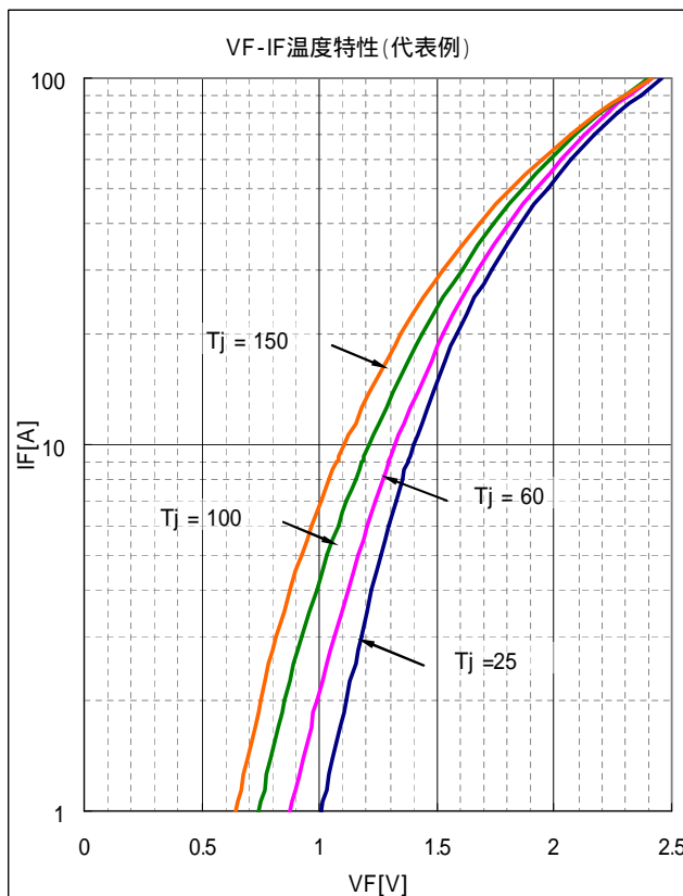
VF-IF・VR-IR 共に、一素子当たりの特性を示す。
