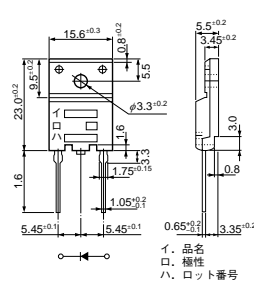
・No. 21 TO3PF2Pin
