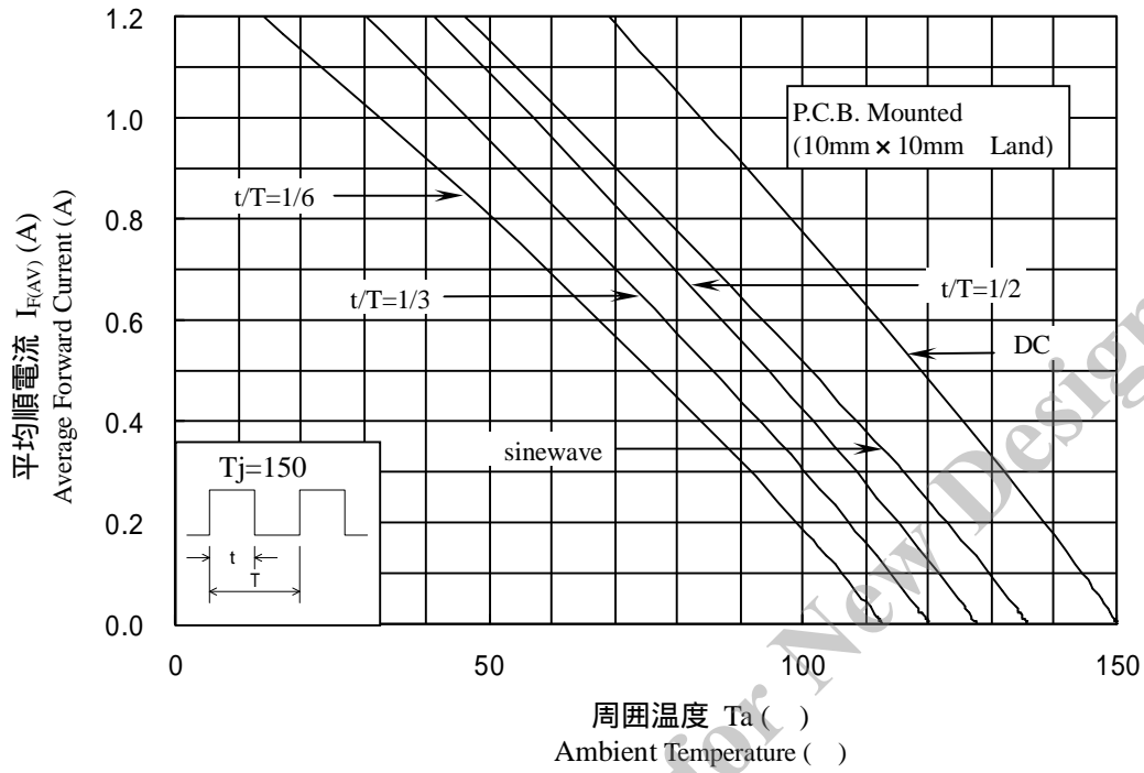
周囲温度 平均順電流 Ta - I F(AV)
