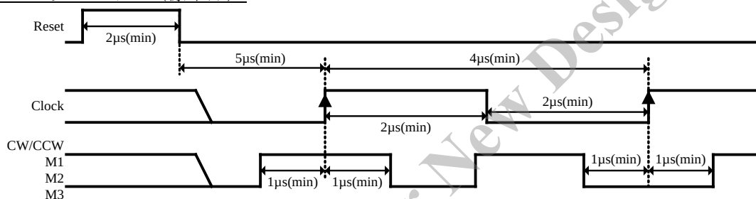
図 11-1 入力信号のタイミング
