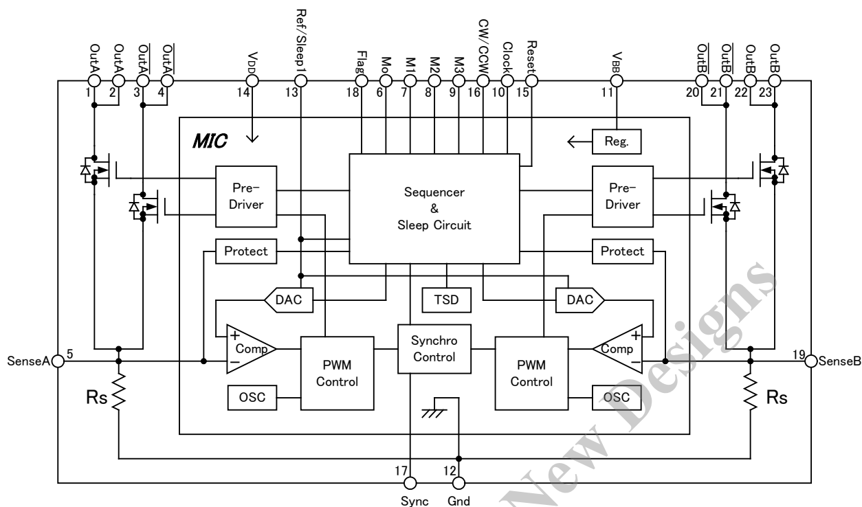
図 7-2 SLA7078MS : \mu ステップ対応品
