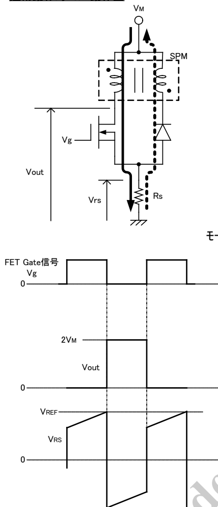
図 14-7 負荷オープン保護動作
