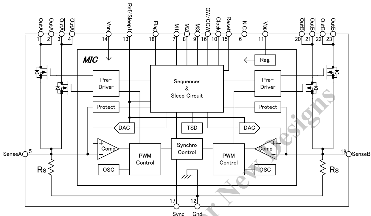
図 7-1 SLA7072MS、SLA7073MS : Full/Half ステップ対応品
