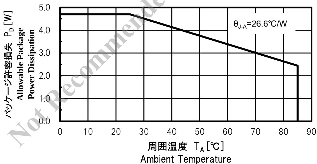
図 5-1 減定格図
