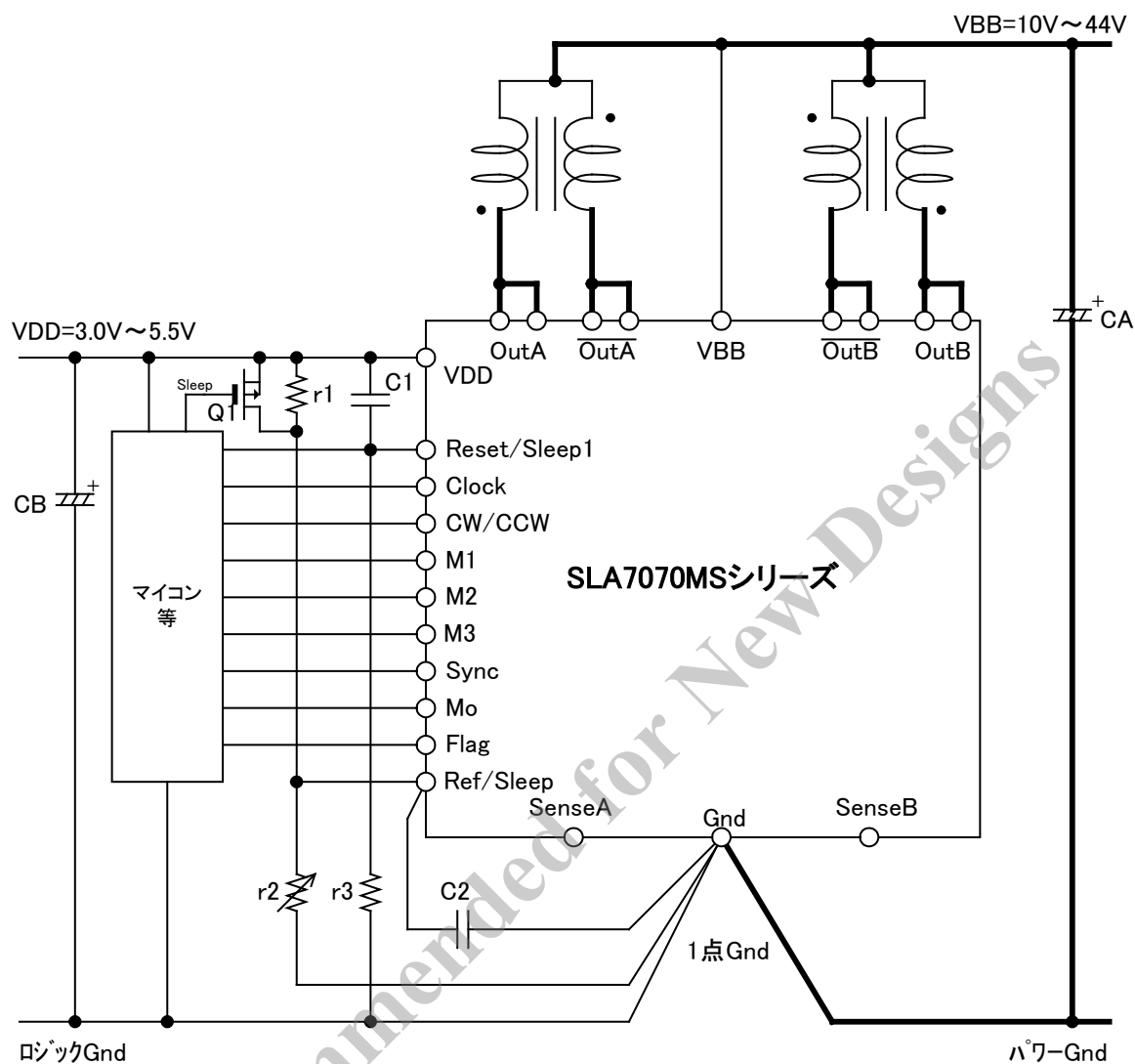
図 8-1 代表例： \mu ステップ対応品
