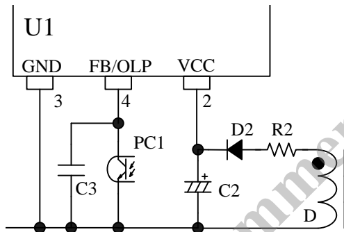
図 9-12 FB/OLP 端子周辺回路
