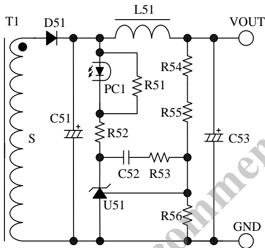
図 10-3 二次側シャントレギュレータ(U51)の周辺回路
