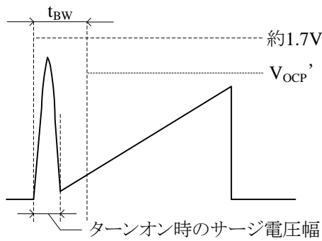
図 9-9 S/OCP 端子電圧波形
