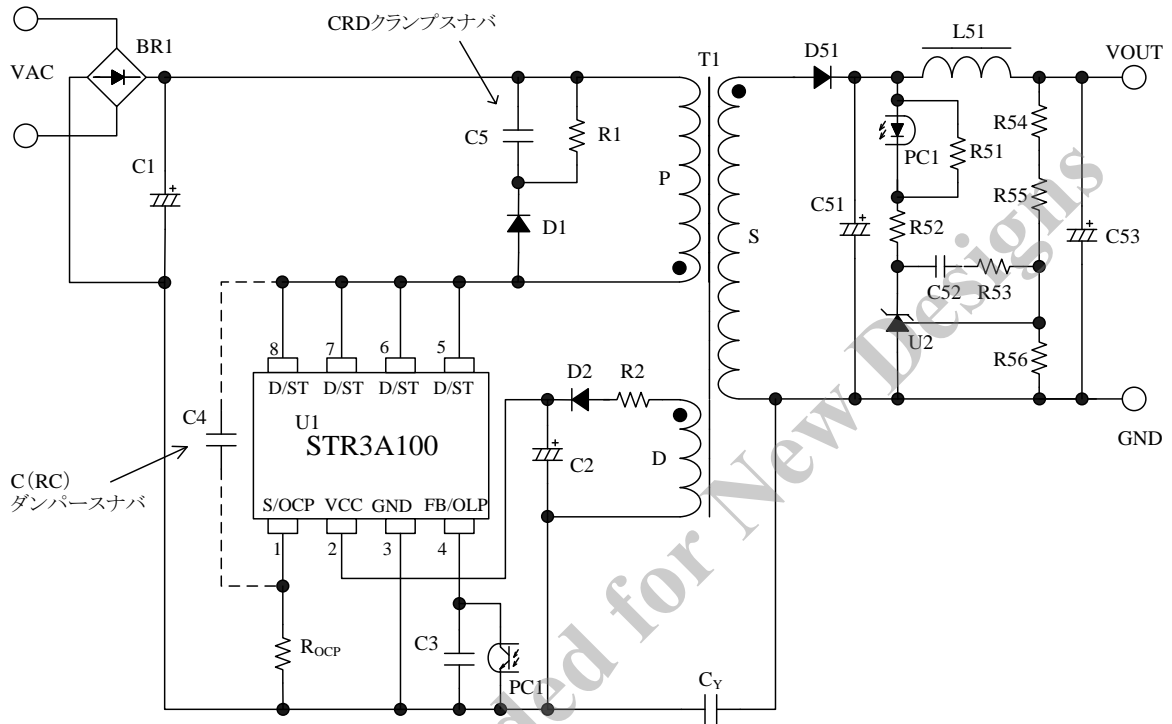
図 6-1 応用回路例
