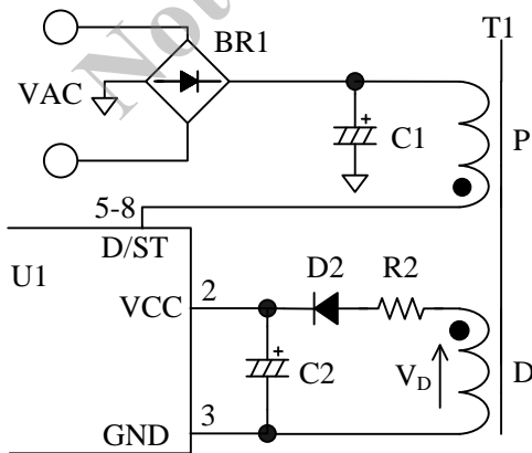
図 9-1 VCC 端子周辺回路
