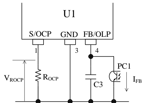
図 9-5 FB/OLP 端子周辺回路
