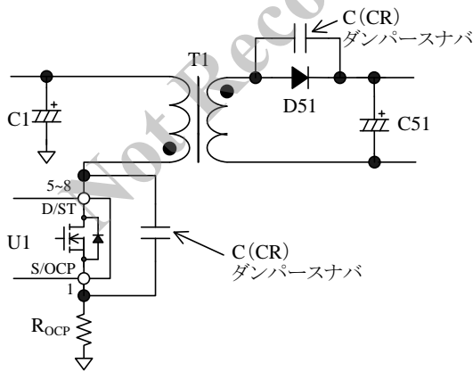
図 9-10 ダンパースナバ
