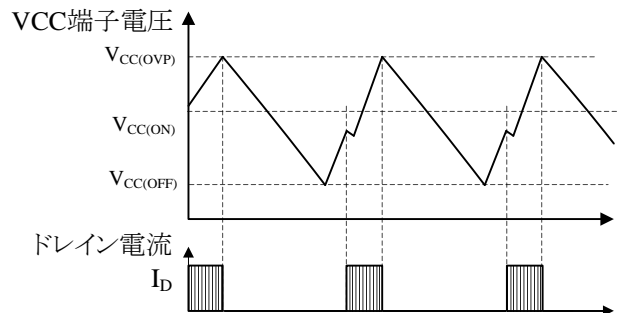
図 9-14 OVP 動作波形
