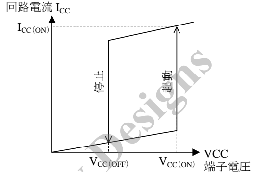
図 9-2 VCC 端子電圧と回路電流 I_{CC}
