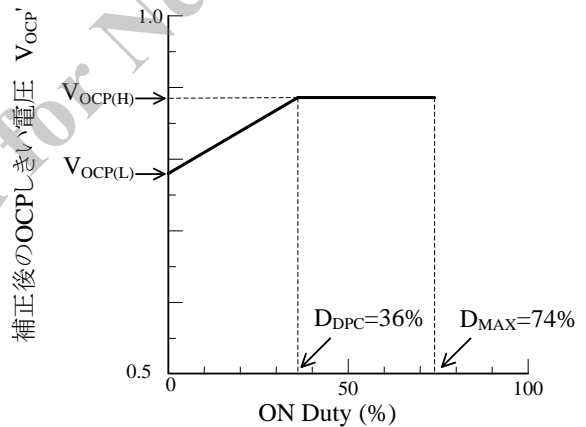
図 9-11 オンデューティと補正後の V_{OCP}
