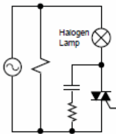
ヒーター温度制御
