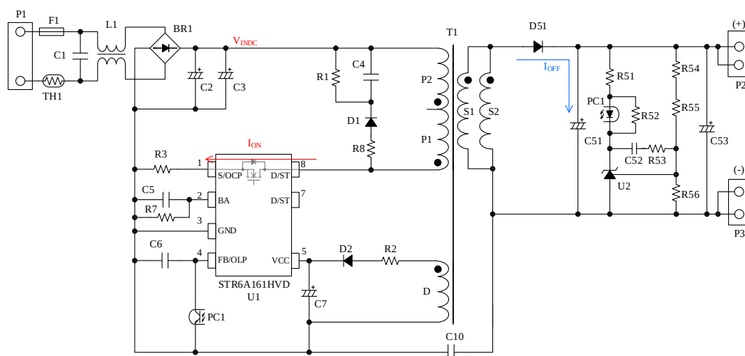
図 6-1 回路図
