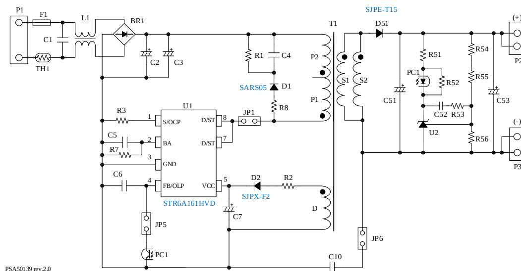
图 5-1 回路图
