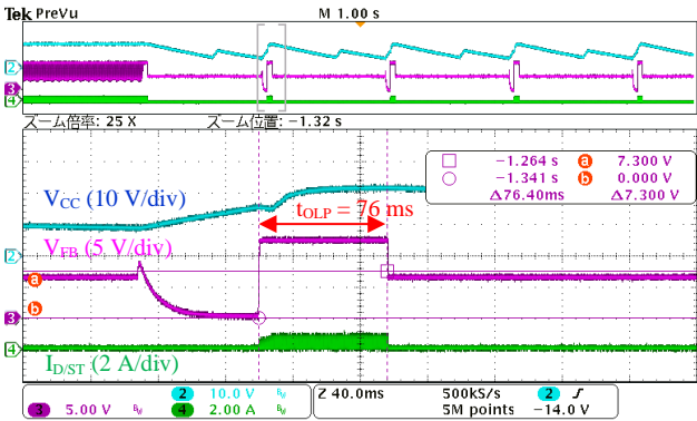
图 9-25 OCP、OLP 动作波形 (图 9-23 A 部扩大)
