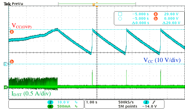
图 9-28 OVP 动作波形 ( V_{IN} = 265 \text{ VAC} 、 I_O = 0 \text{ A} )
