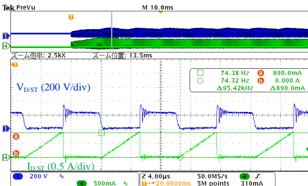
图 9-3 启动时的动作波形 (图 9-1 A 部分扩大)
