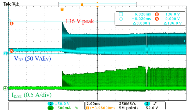
图 9-10 启动时 D2 动作波形 ( V_{IN} = 265 \text{ VAC} 、 I_O = 1.0 \text{ A} )
