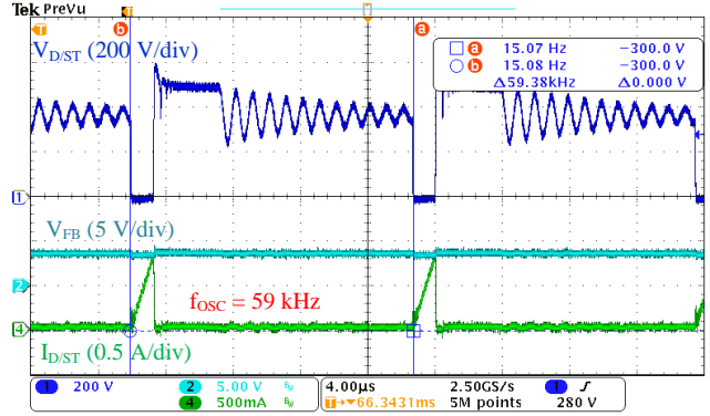
图 9-14 轻载动作波形
