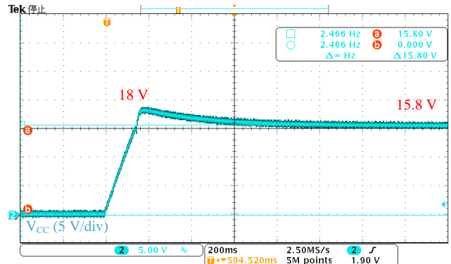
图 9-8 启动时 VCC 引脚电压波形 ( V_{IN} = 265 \text{ VAC} 、 I_O = 0 \text{ A} )
