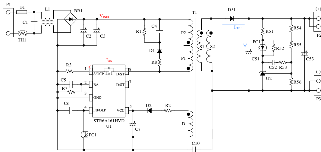
图 6-1 电路图
