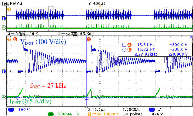
图 9-17 启动时动作波形 (图 9-17 A 部扩大)
