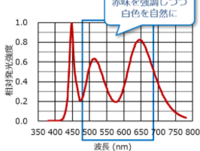
スペクトル
