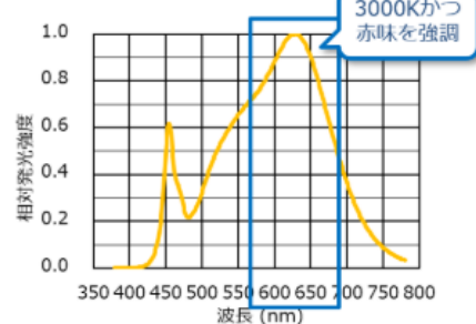
スペクトル
