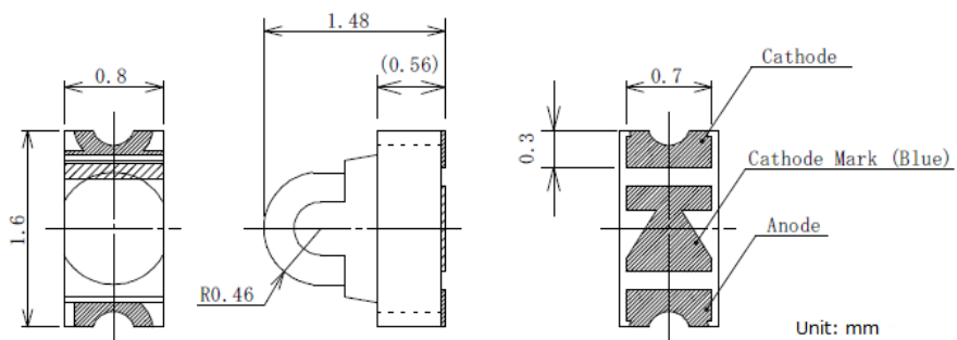
L×W×H : 1.6×0.8×1.5 (ドームタイプ)
