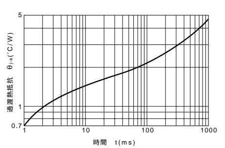
θj-a-t特性
