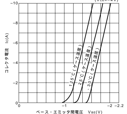
I C -V BE 温度特性 (代表例)
