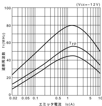
f r -I E 特性 (代表例)
