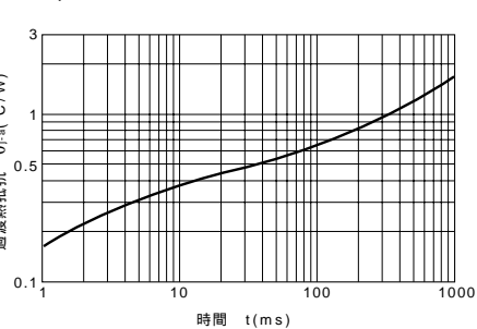
θ j-a -t特性
