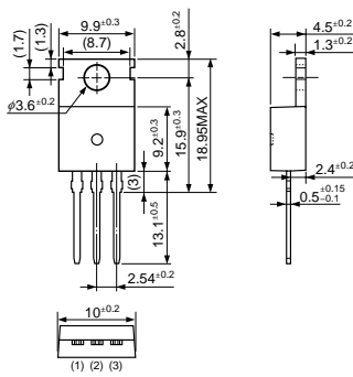
・ TO-220
