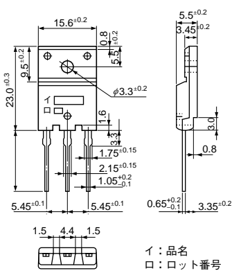
・ TO-3PF
