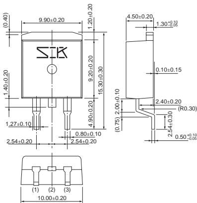
・ TO-263
