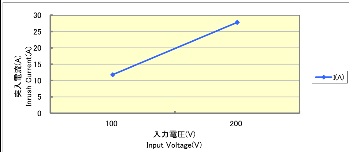
図3 突入電流特性(入力電圧に対して) Fig.3 Inrush Current Characteristics (vs Input Voltage)
