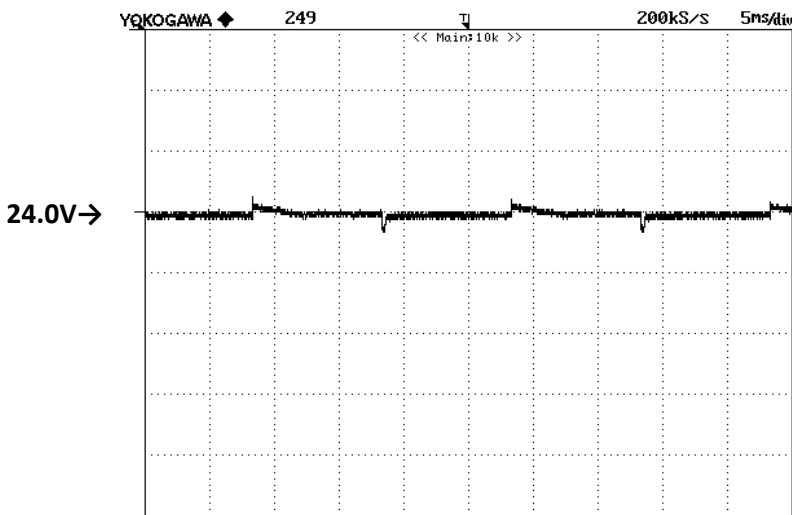
図12 タイミング時の負荷波形 Fig.12 Dynamic Load Waveform
