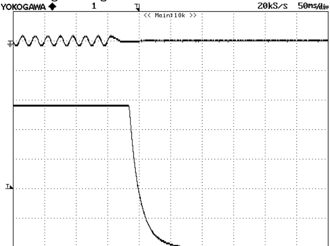
図14 出力電圧立下り波形 Fig.14 Output Voltage Falling Waveform
