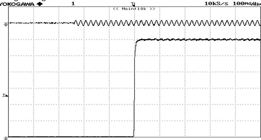
図14 出力電圧立上り波形 Fig.14 Output Voltage Rising Waveform
