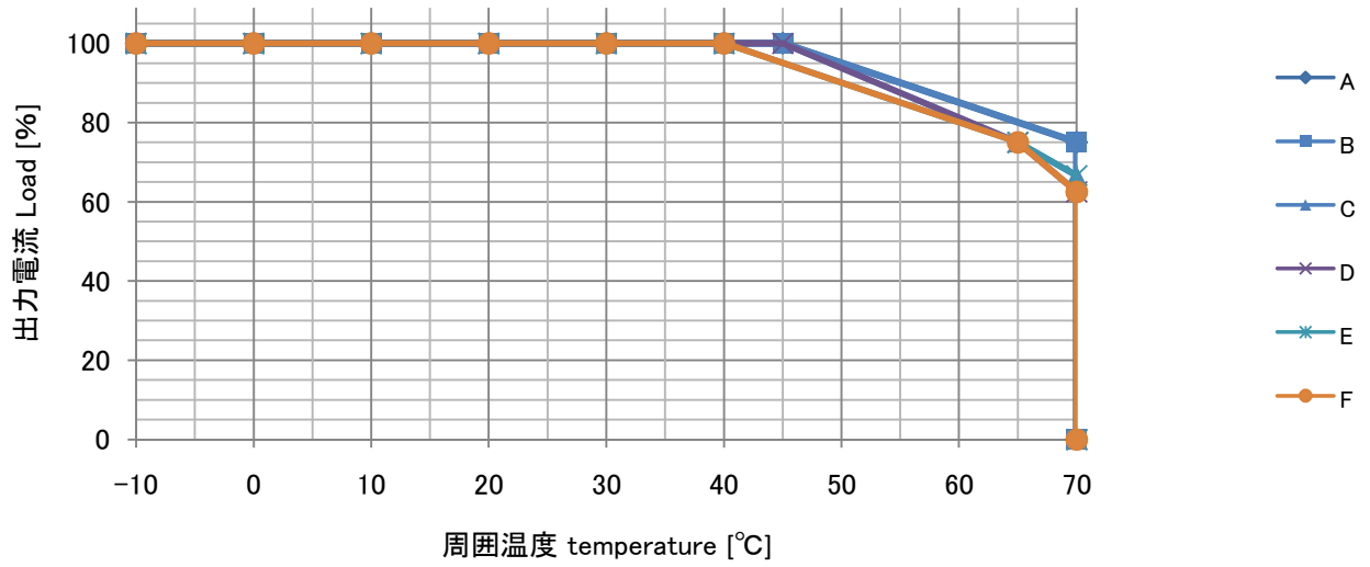
周囲温度によるデレーティングカーブ(カバー無し)
