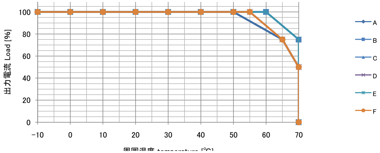
周囲温度によるデレーティングカーブ(カバーあり)
