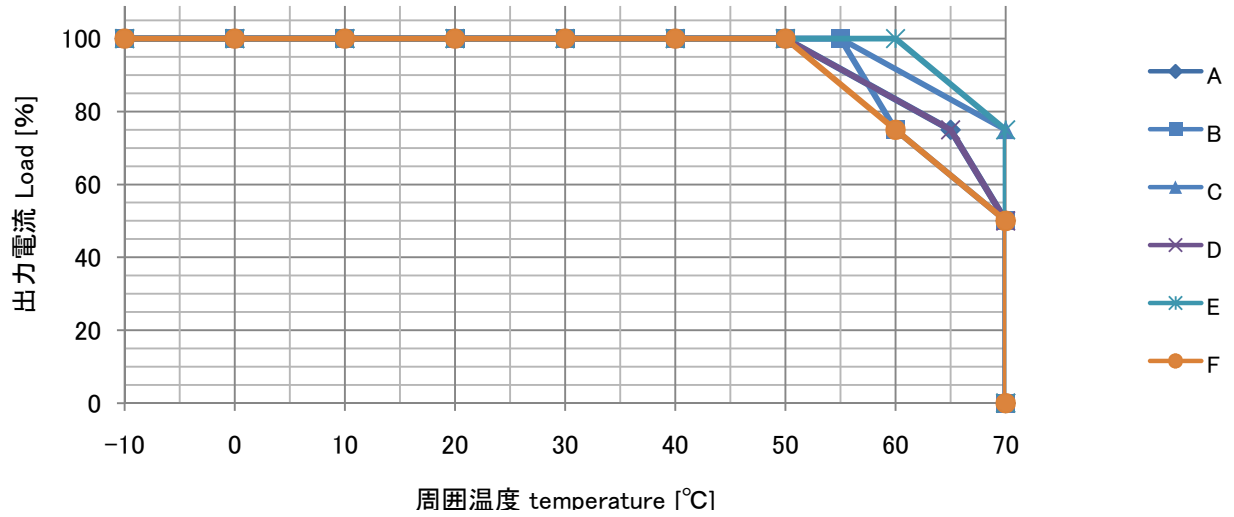
周囲温度によるデレーティングカーブ(カバー無し)
