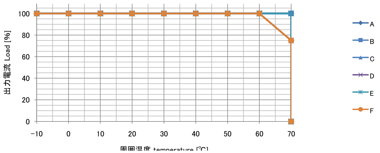
周囲温度によるデレーティングカーブ(シャーシカバーあり)
