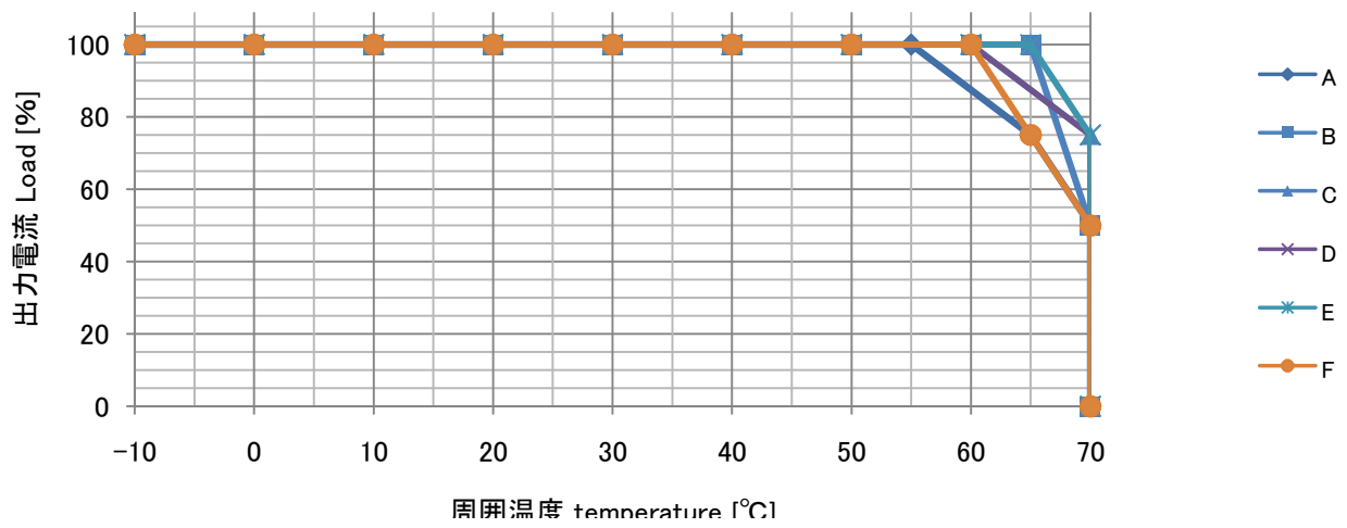
周囲温度によるデレーティングカーブ(カバー無し)
