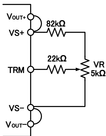
接続図
