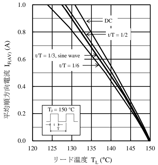
図3 I_{F(AV)} - T_L 代表特性 ( V_R = 400 \text{ V} )
