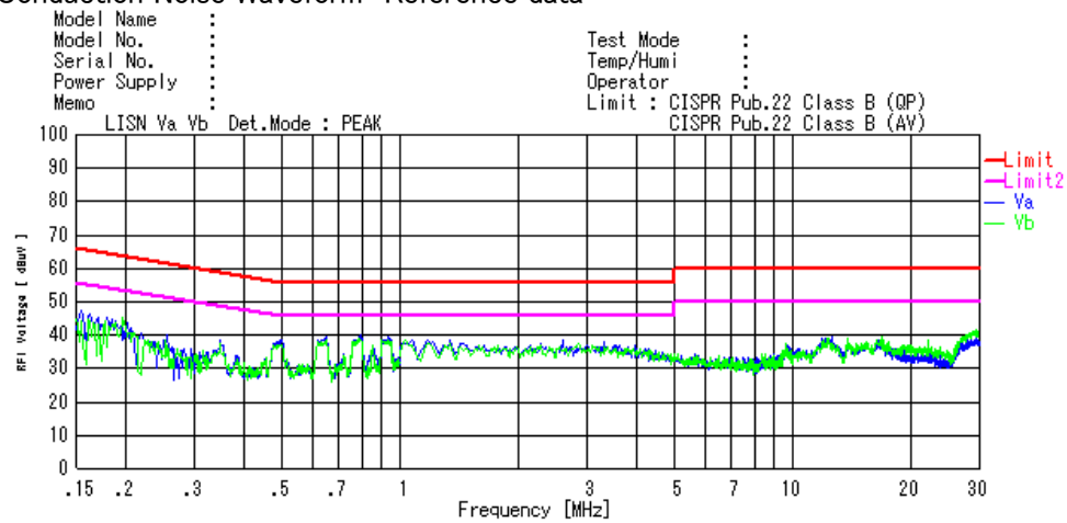
Fig.19 雑音端子電圧波形 参考データ Fig.19 Conduction Noise Waveform Reference data
