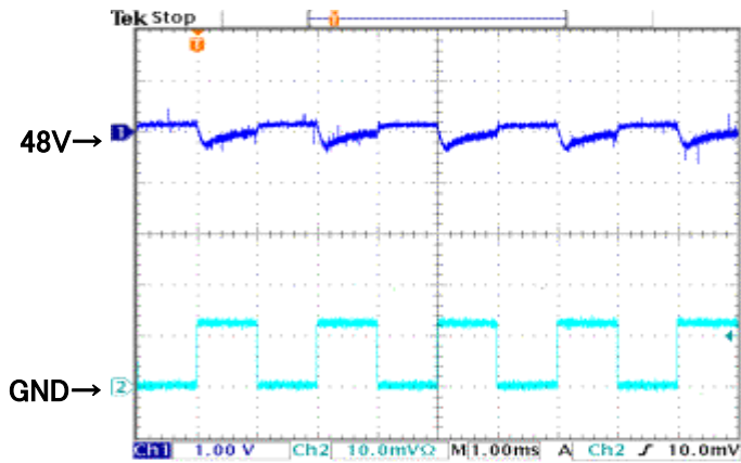
図13 ダイナミック時の負荷波形 Fig.13 Dynamic Load Waveform
