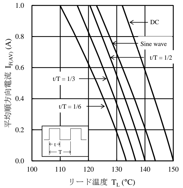
図3 I_{F(AV)} - T_L 特性 ( T_J = 150 °C、 V_R = 1000 V)
