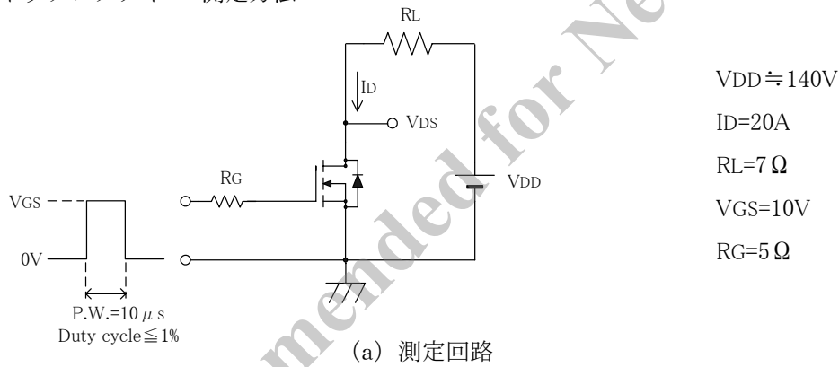
図2 スイッチングタイム 測定方法
