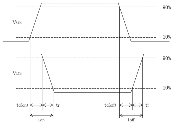
(b) 出力波形
