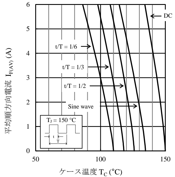
図 2 I_{F(AV)} - T_C 代表特性 ( V_R = 60 V )
