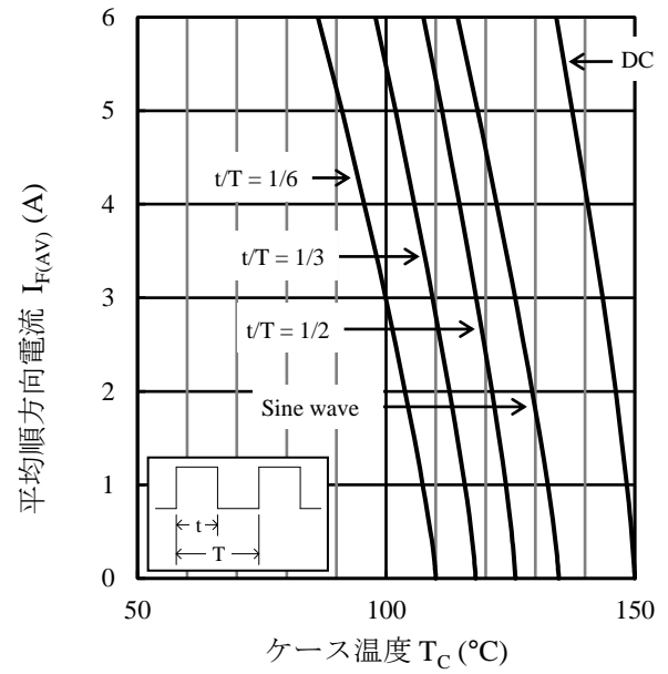
図 2 I_{F(AV)} - T_C 特性 ( T_J = 150 °C、 V_R = 60 V)
