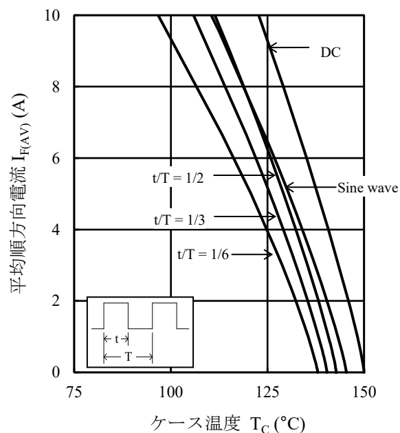
図2 I_{F(AV)} - T_C 特性 ( T_J = 150\text{ }^{\circ}\text{C} 、 V_R = 100\text{ V} )
