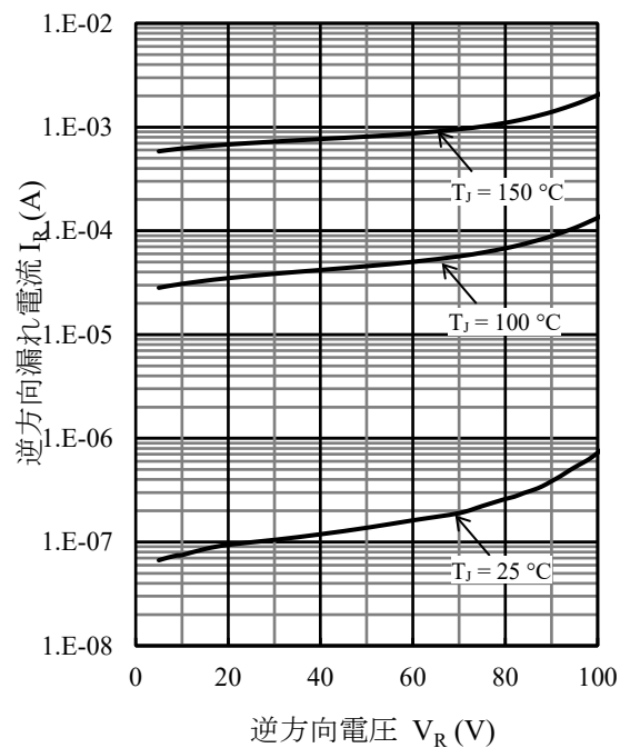
図6 I_R - V_R 代表特性
