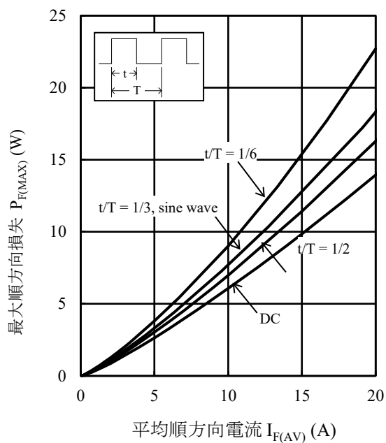
図 3 P_{F(MAX)} - I_{F(AV)} 特性 ( T_J = 150 °C)
