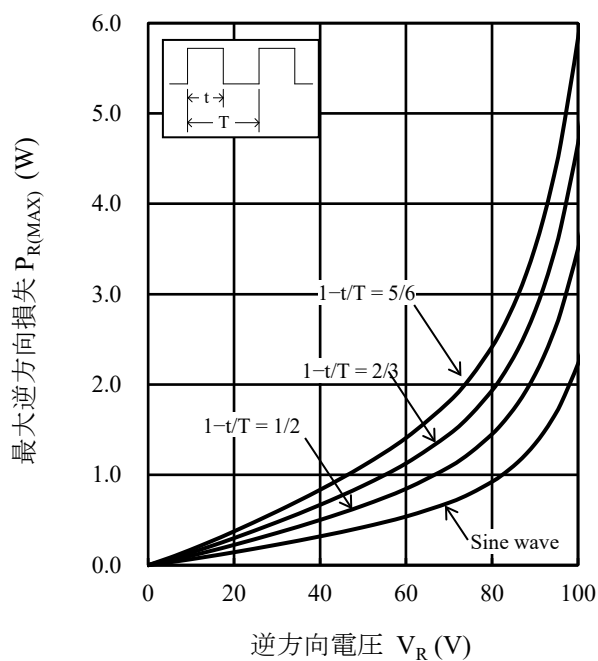
図 4 P_{R(MAX)} - V_R 特性 ( T_J = 150 °C)
