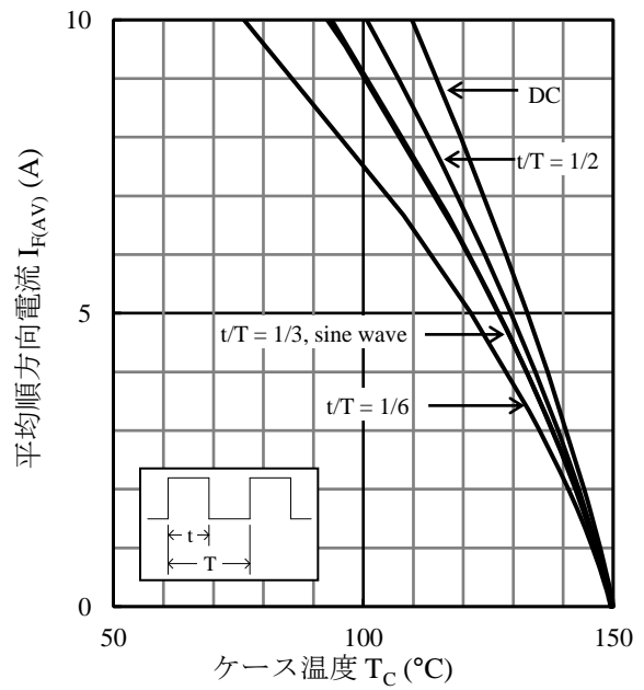
図2 I_{F(AV)} - T_C 特性 ( T_J = 150 °C、 V_R = 400 V)
