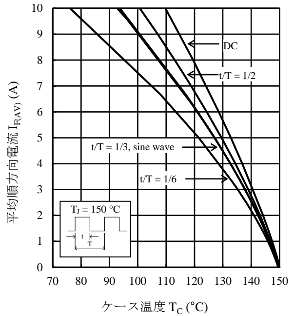
図 2 I_{F(AV)} - T_C 代表特性 ( V_R = 400 \text{ V} )
