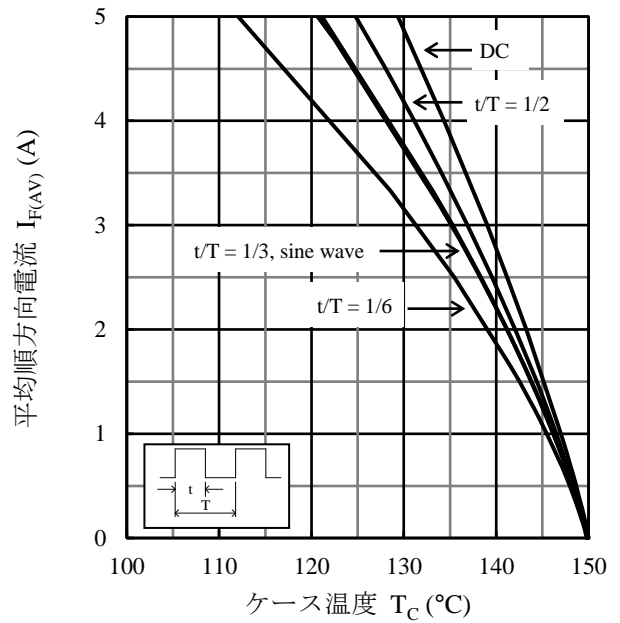
図2 I_{F(AV)} - T_C 特性 ( T_J = 150\text{ }^\circ\text{C} , V_R = 300\text{ V} )
