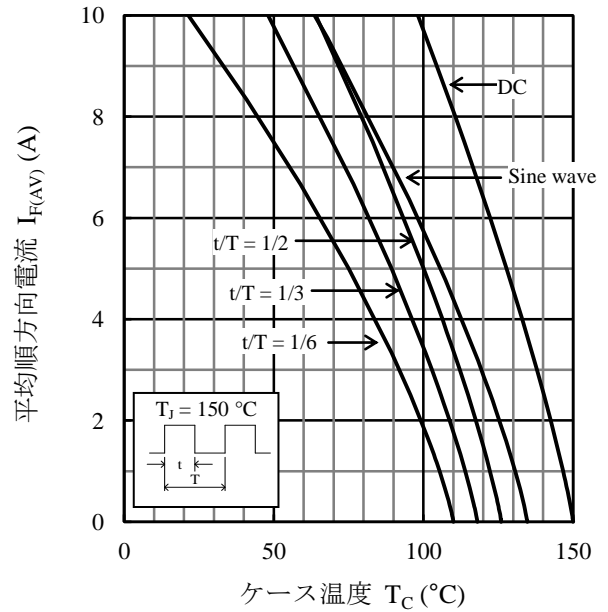
図 2 I_{F(AV)} - T_C 代表特性 ( V_R = 400 V)
