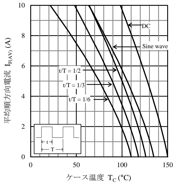
図2 I_{F(AV)} - T_C 特性 ( T_J = 150 °C、 V_R = 400 V)
