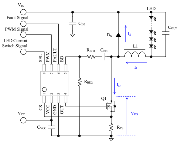
図 9-1 LC5910S を用いた LED 駆動回路例
