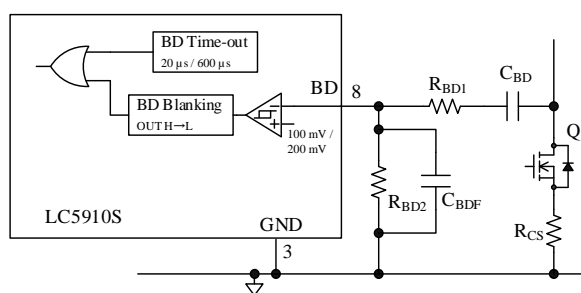
図 9-4 BD 端子接続
