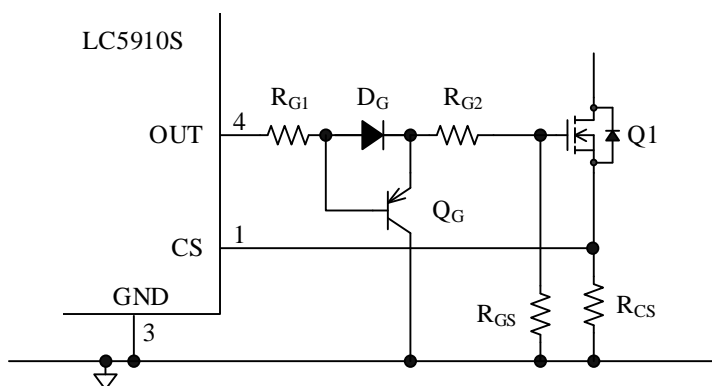
図 9-7 OUT 端子周辺回路例(2)
