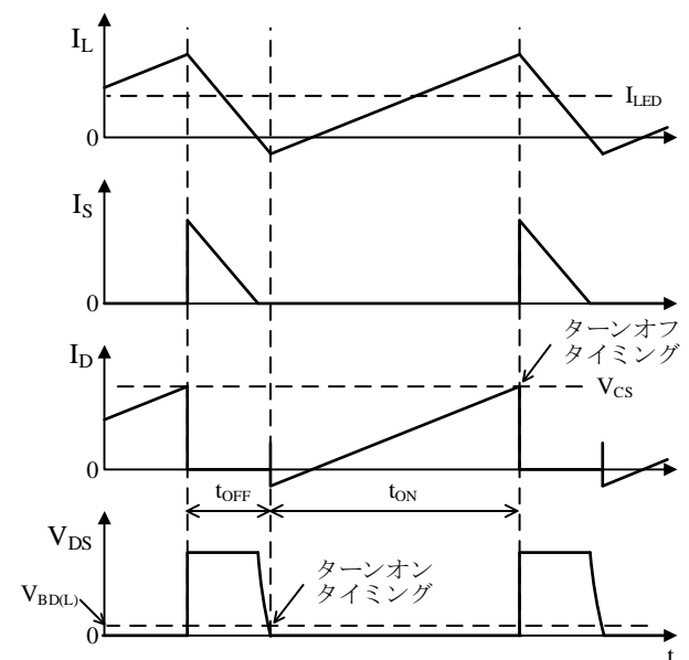
図 9-2 LC5910S の CRM 制御
