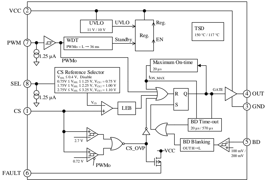
図 4-1 LC5910S ブロックダイアグラム
