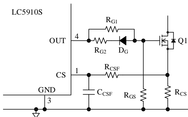
図 9-8 CS 端子の RC フィルタ
