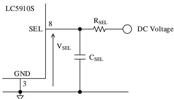
図 9-3 SEL 端子の RC フィルタ
