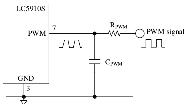
図 9-5 PWM 端子の RC フィルタ
