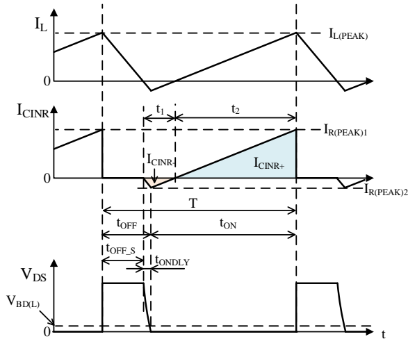
図 10-2 C IN リップル電流（ワースト条件）
