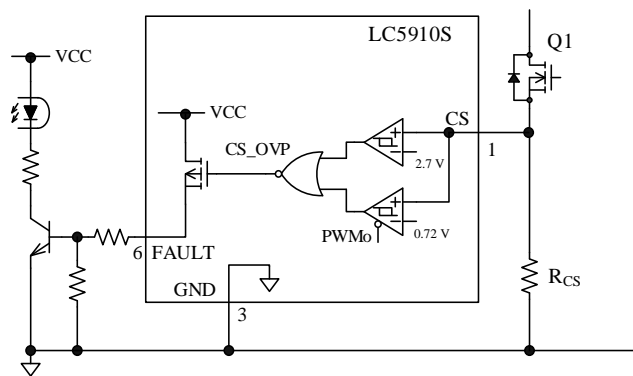
図 9-9 FAULT 端子周辺回路
