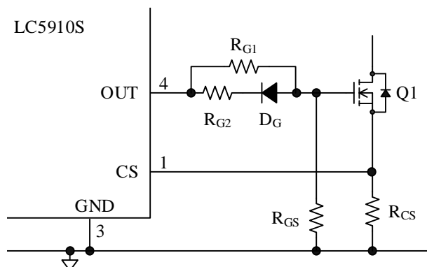
図 9-6 OUT 端子周辺回路例(1)
