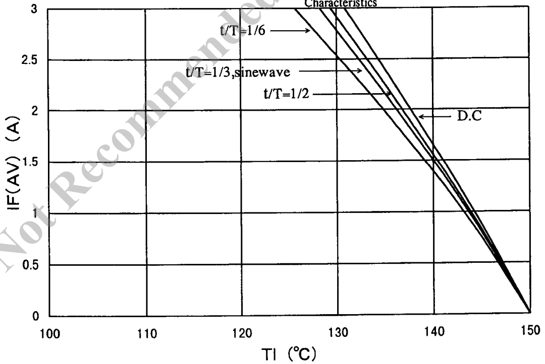
TI - IF(AV) 特性 Characteristics
