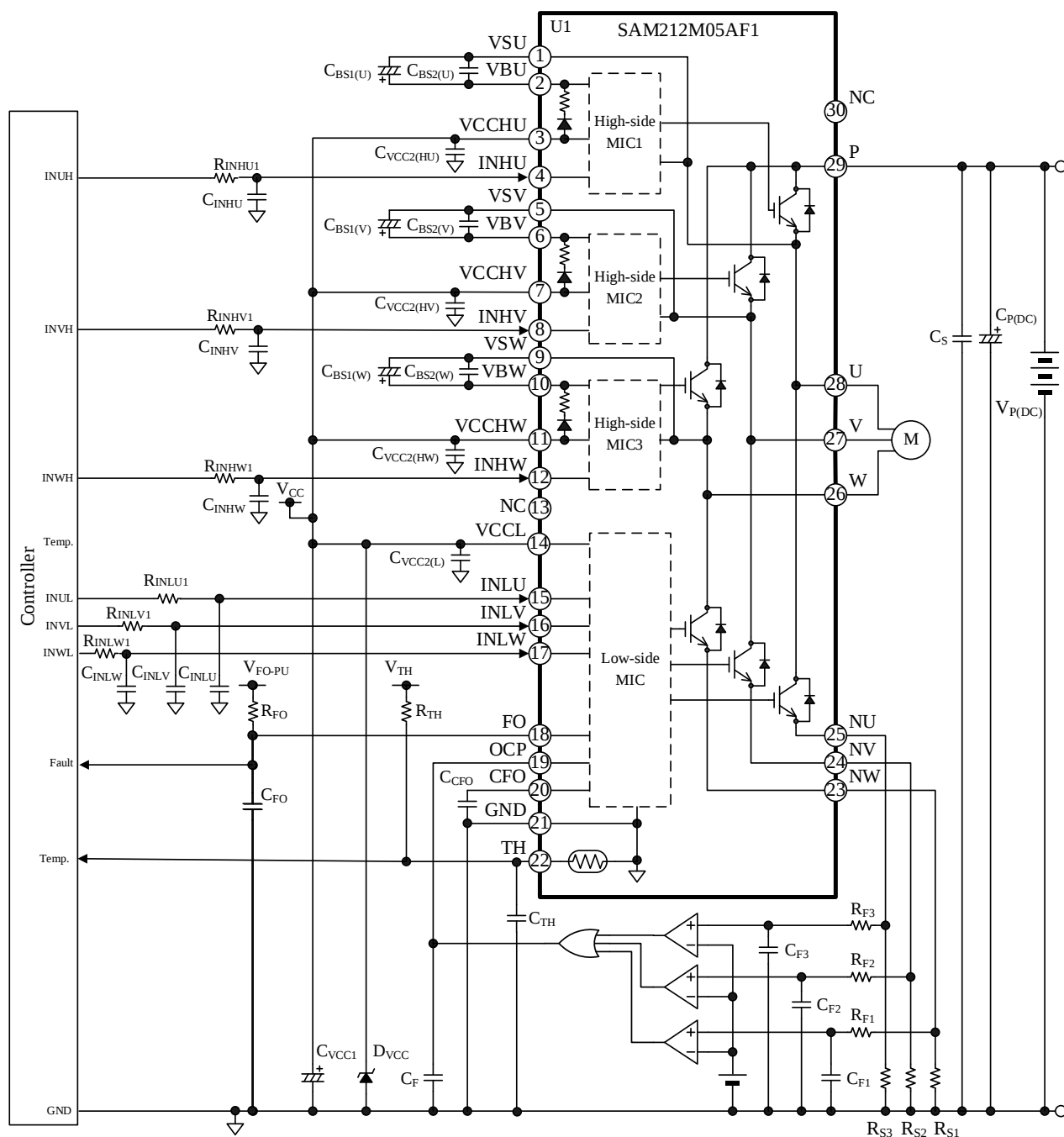
図 10-2 応用回路例 (3 シェント検出方式)
