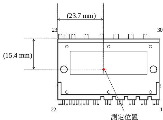
図 2-1 ケース温度測定位置
