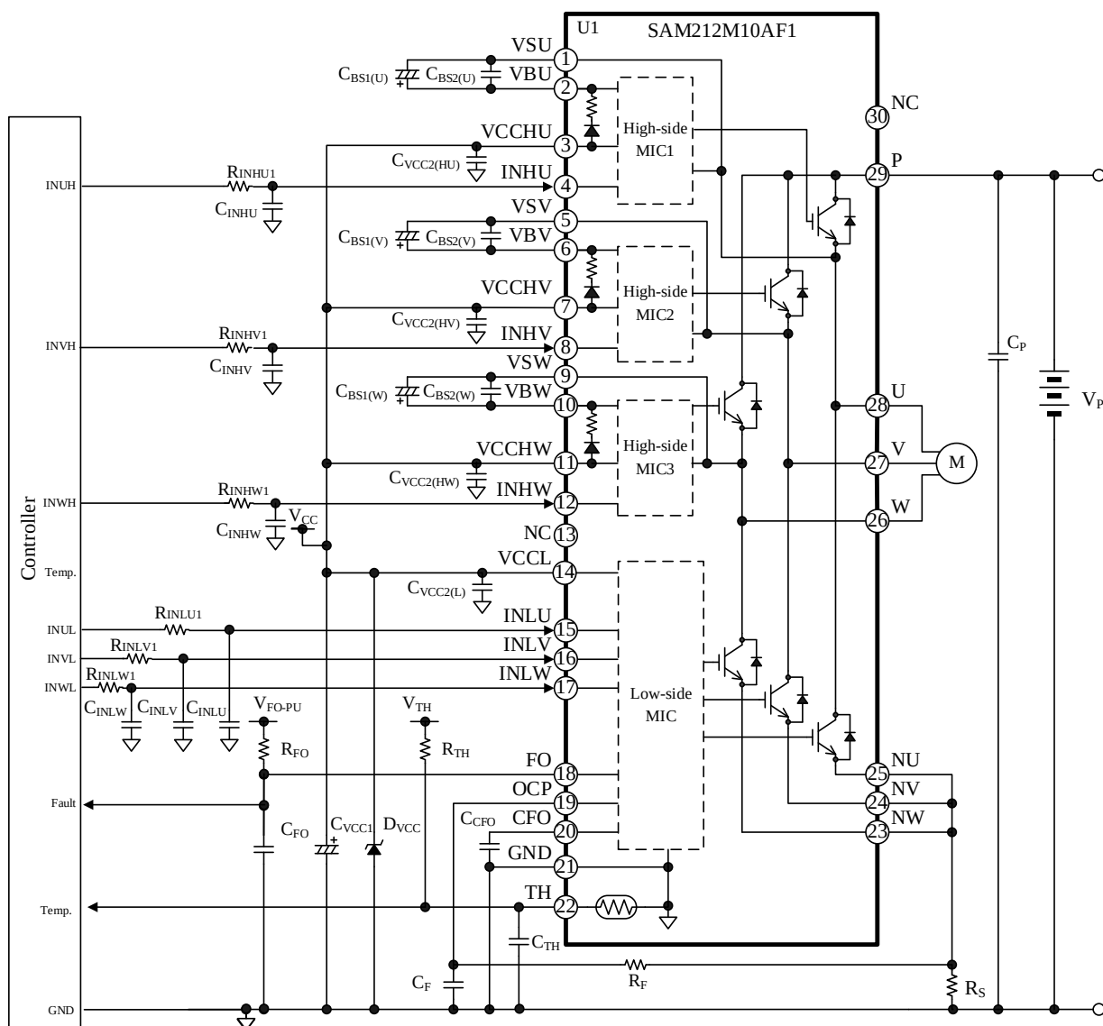
図 10-1 応用回路例 (1 シャント検出方式)
