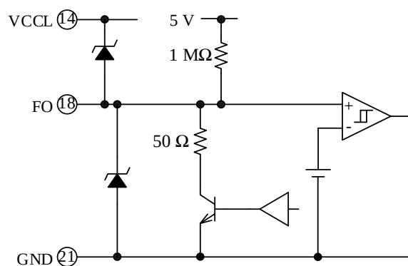
図 8-3 FO 端子内部回路図
