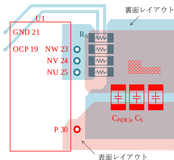
図 14-2 C_S 周辺のレイアウト例（両面基板）
