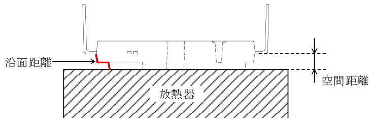
図 6-1 絶縁距離測定位置
