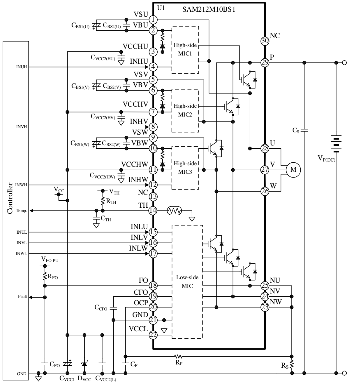
図 10-1 応用回路例 (1 シヤント検出方式)
