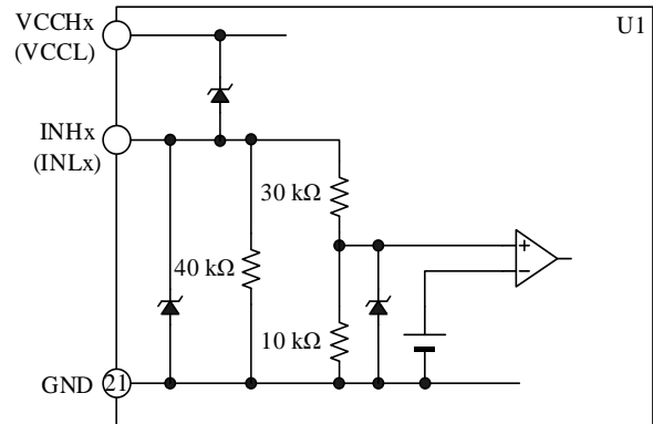
図 13-5 INHX 端子、INLX 端子の内部回路図
