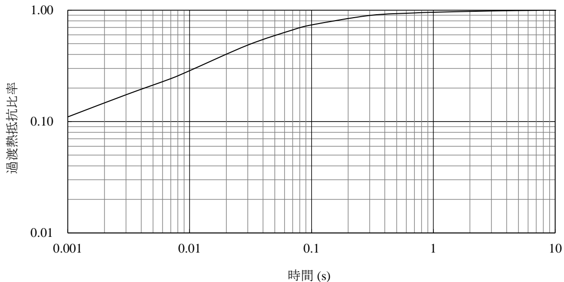
図 16-1 過渡熱抵抗比率
