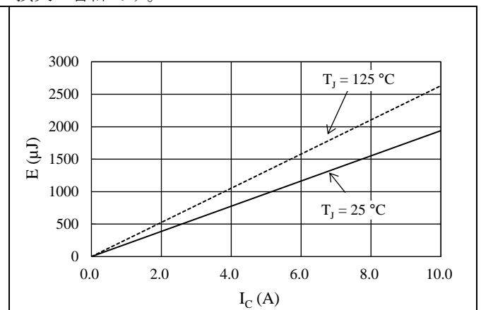
図 16-5 ローサイドスイッチング損失特性
