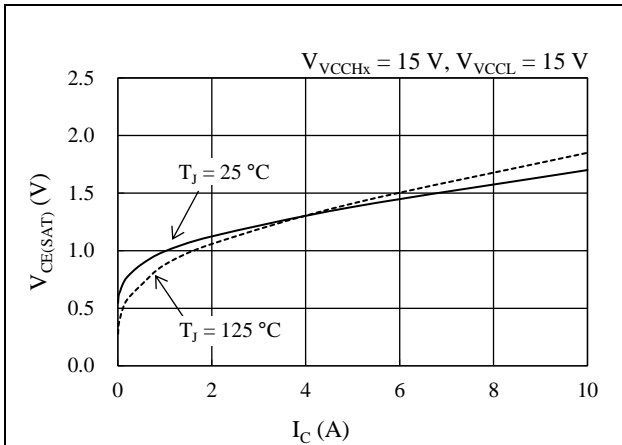
図 16-2 IGBT V_{CE(SAT)} - I_C 特性
