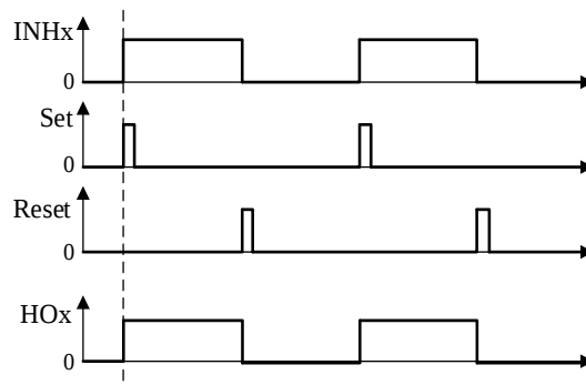
図 13-3 レベルシフト部動作波形
