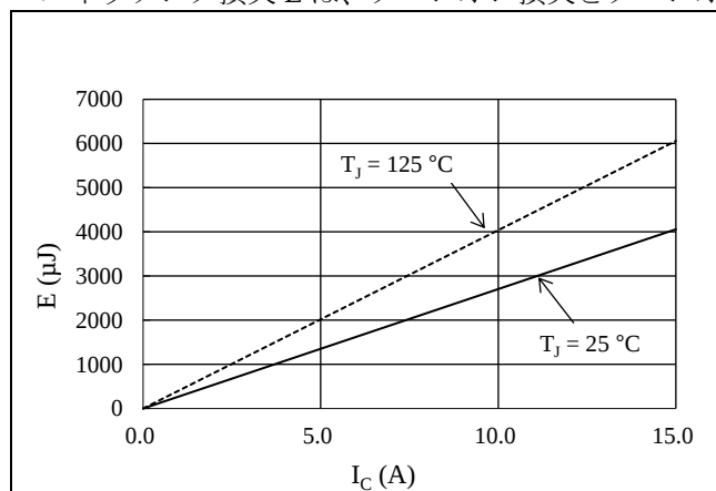
図 16-4 ハイサイドスイッチング損失特性
