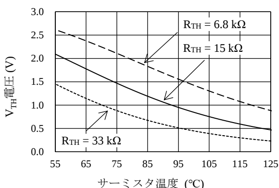
図 13-10 V_{TH} 電圧 - サーマスタ温度特性 ( V_{TH\_PU} = 3.3\text{ V} )
