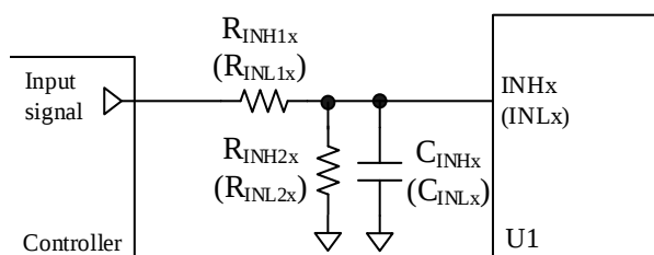
図 13-6 INHx 端子、INLx 端子のフィルタ回路
