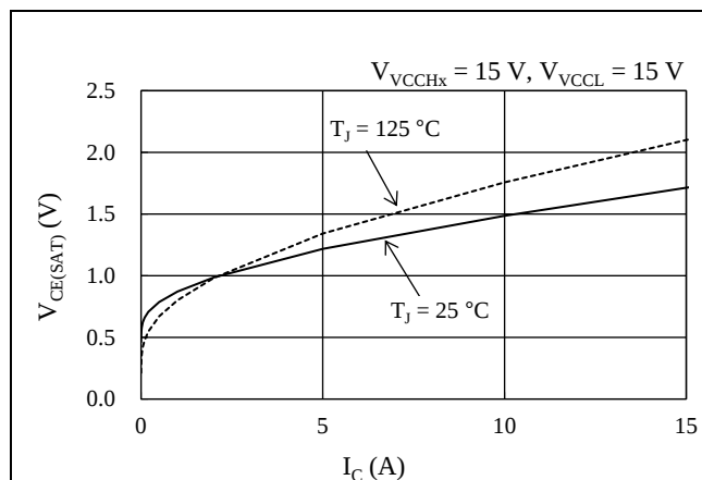
図 16-2 IGBT V_{CE(SAT)} - I_C 特性
