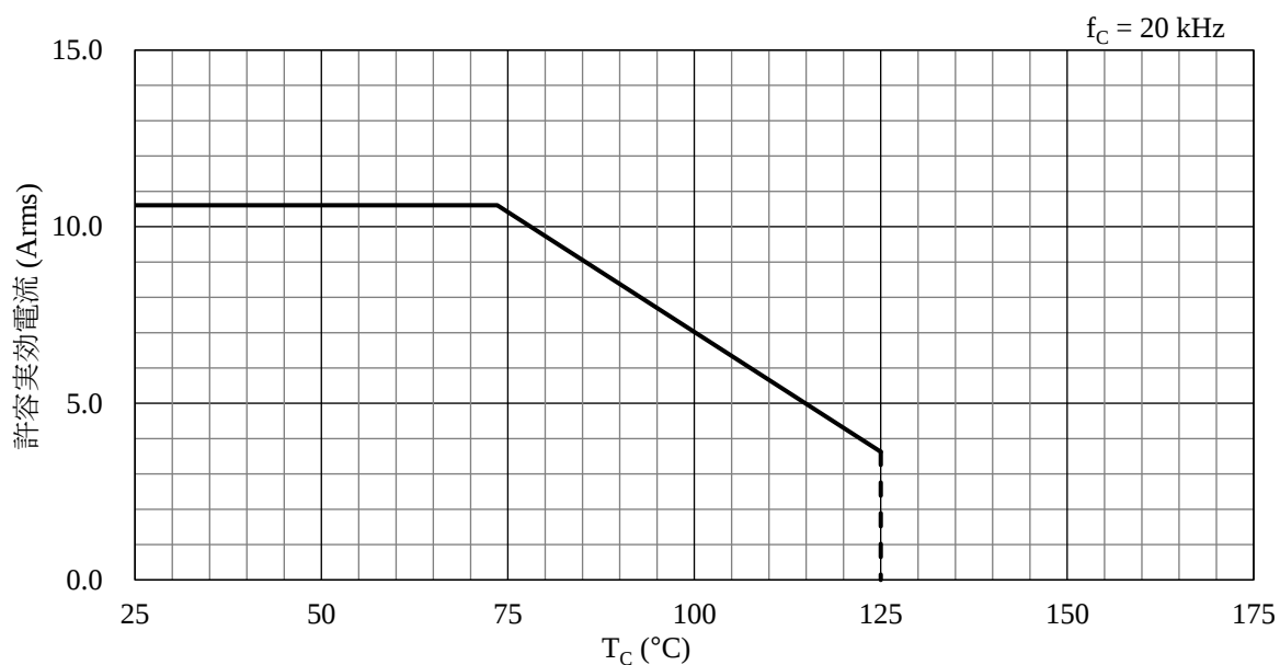
図 16-7 許容電流特性 ( f_C = 20\text{ kHz} )
