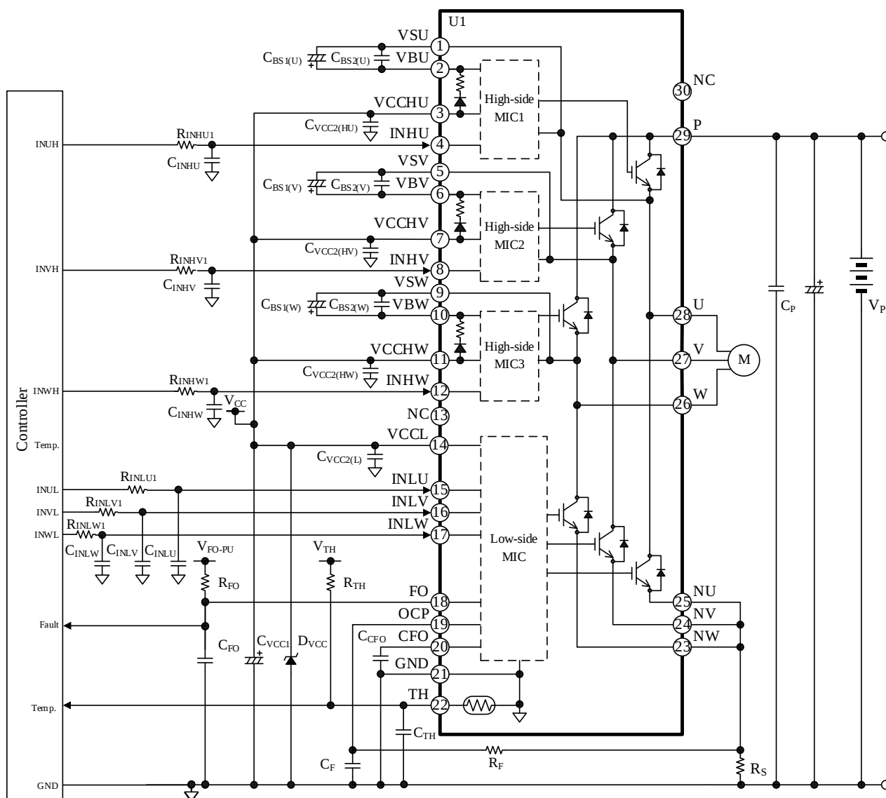
図 10-1 応用回路例 (1 シャント検出方式)
