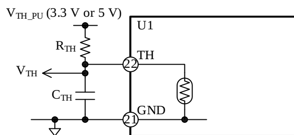
図 13-9 TH 端子の周辺回路と内部回路
