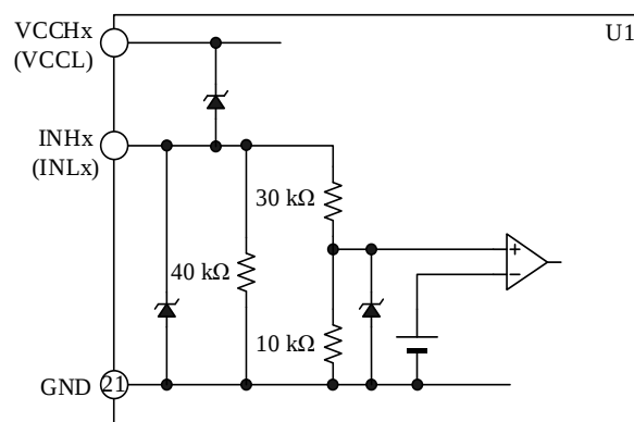
図 13-5 INHx 端子、INLx 端子の内部回路図
