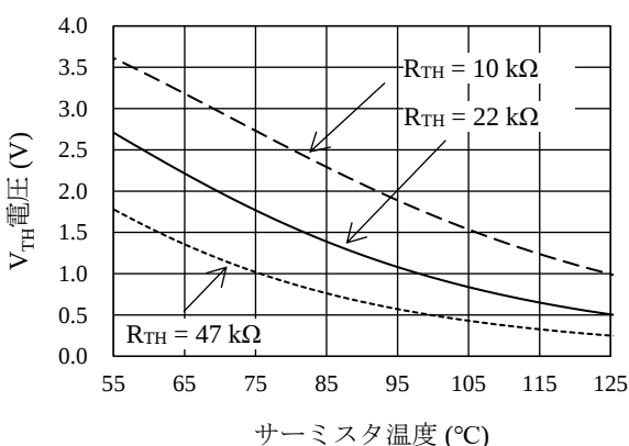
図 13-11 V_{TH} 電圧 - サーマスタ温度特性 ( V_{TH\_PU} = 5.0\text{ V} )
