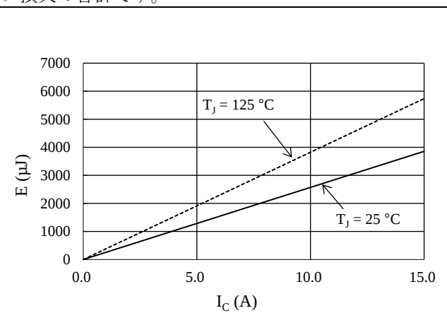
図 16-5 ローサイドスイッチング損失特性
