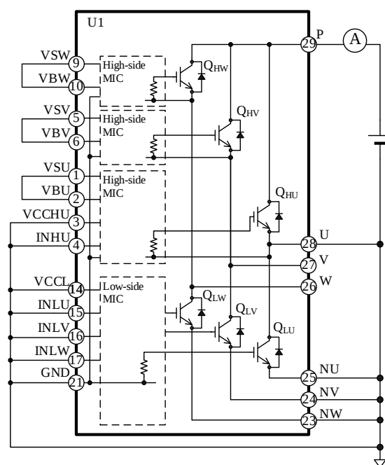
図 14-3 U 相ハイサイド IGBT ( Q_{HU} ) の漏れ電流測定回路
