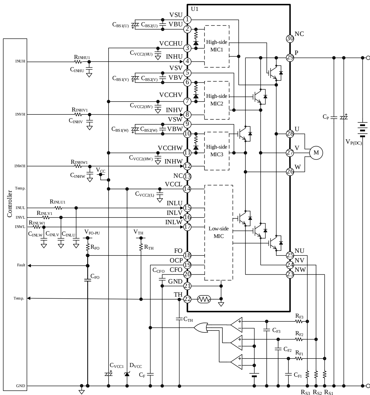
図 10-2 応用回路例 (3 シャント検出方式)
