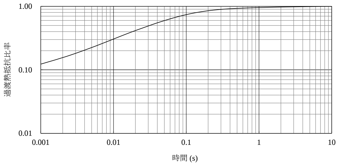
図 16-1 過渡熱抵抗比率
