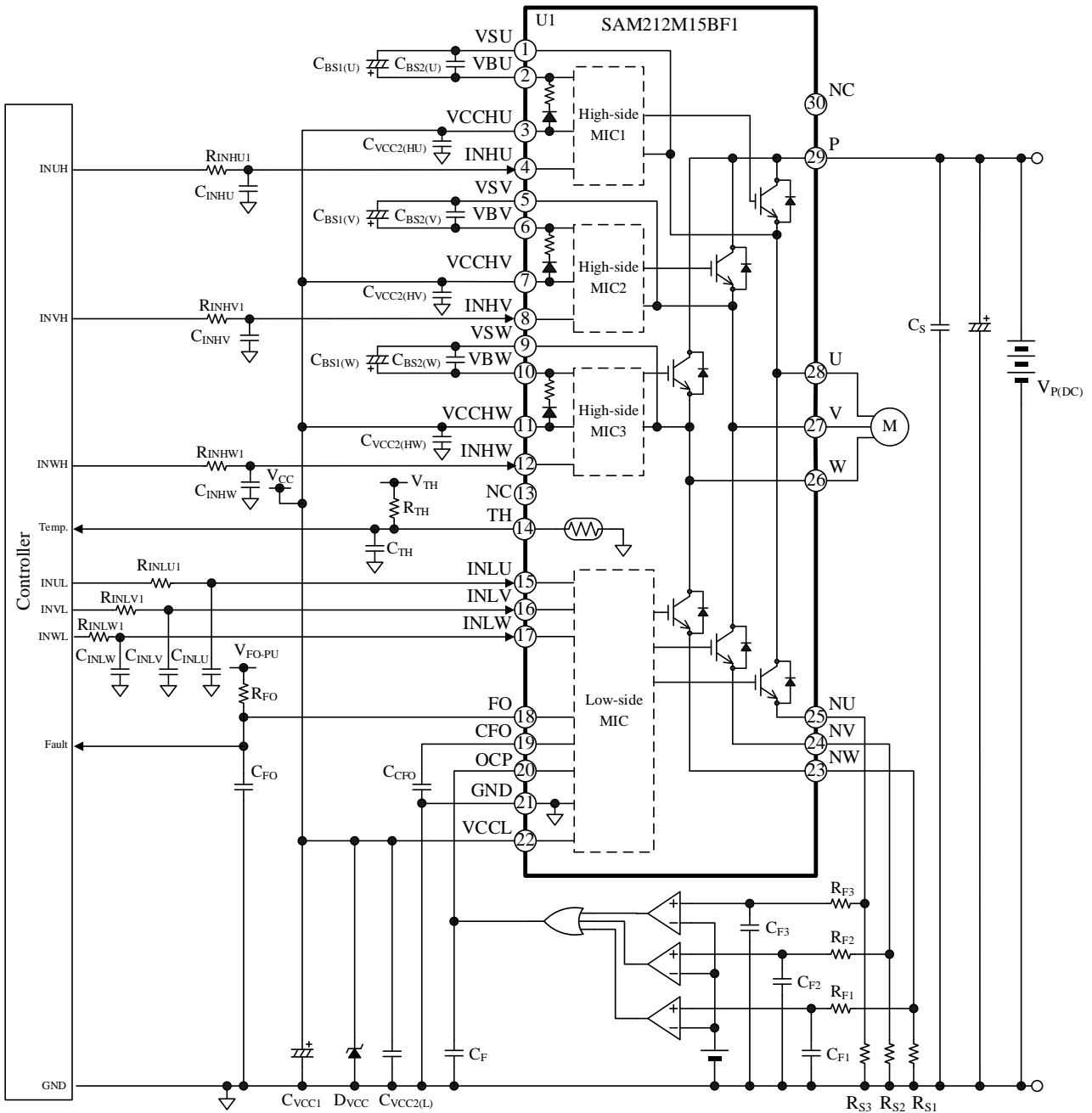
図 10-2 応用回路例 (3 シャント検出方式)
