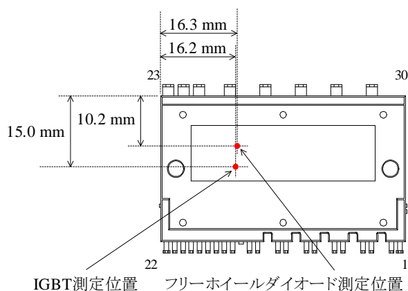
図 4-5 ケース温度測定位置
